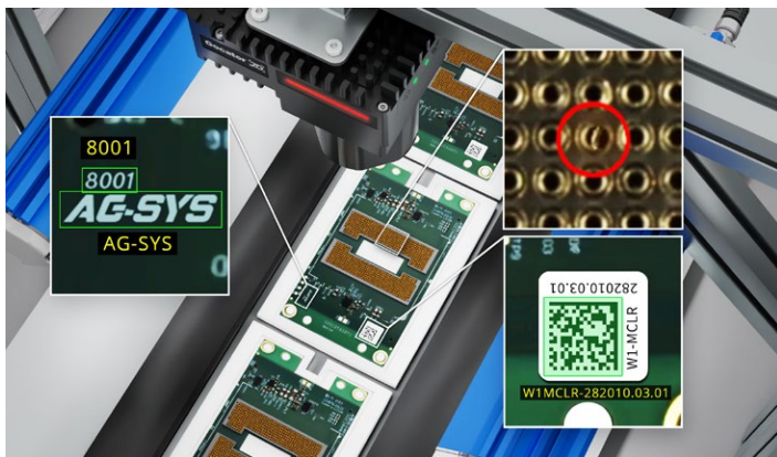
Inspección de sockets de PCB con lectura de código Data Matrix y OCR
